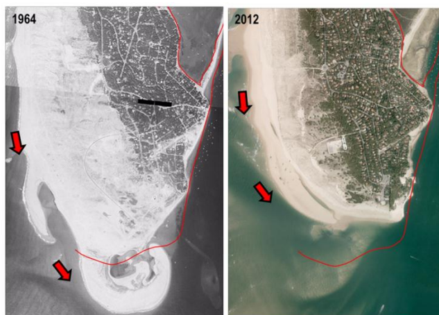
Fig. 8. Représentation schématique du transit de sables en 1964 et 2012
