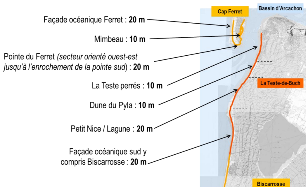
Fig. 12. Valeurs de L_{max} validées par le BRGM (13 jan. 2015)
