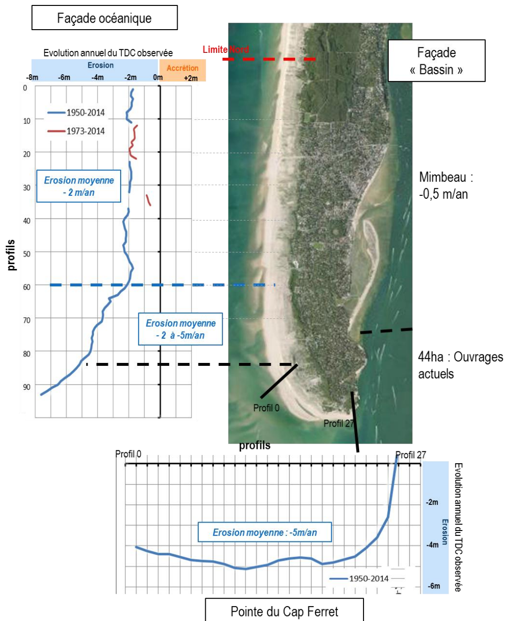
Fig. 11. : Observations du TDC au niveau du Cap Ferret
