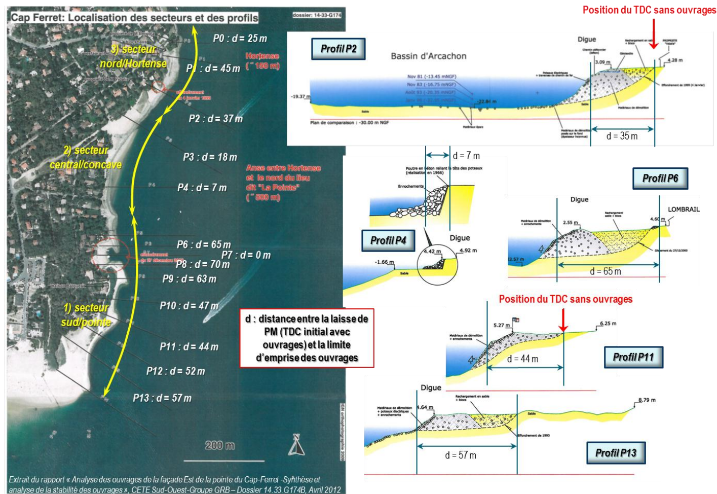
Fig. 4. Analyse des profils des ouvrages du rapport CETE/GRB - 2012
