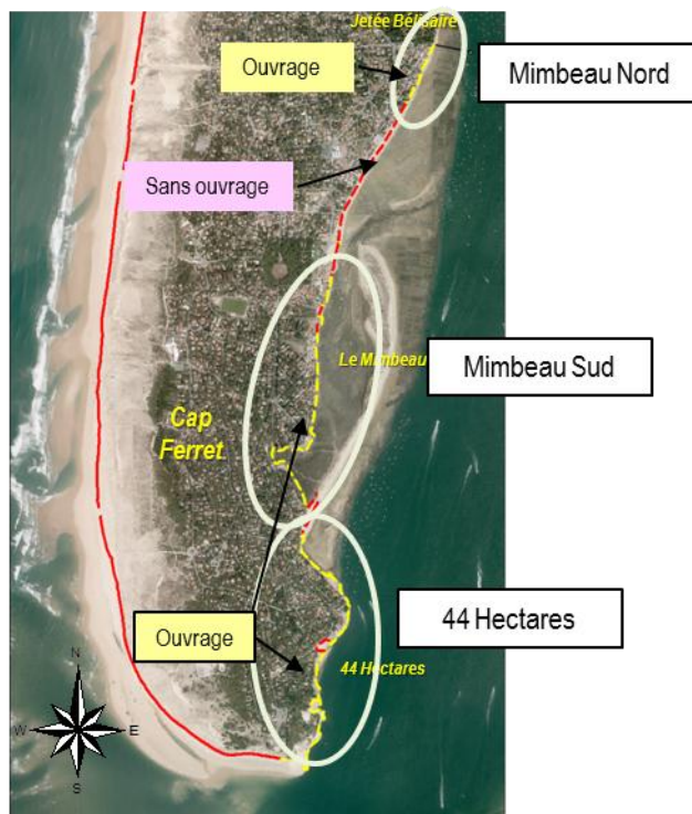
Fig. 3. Secteurs avec ouvrages
